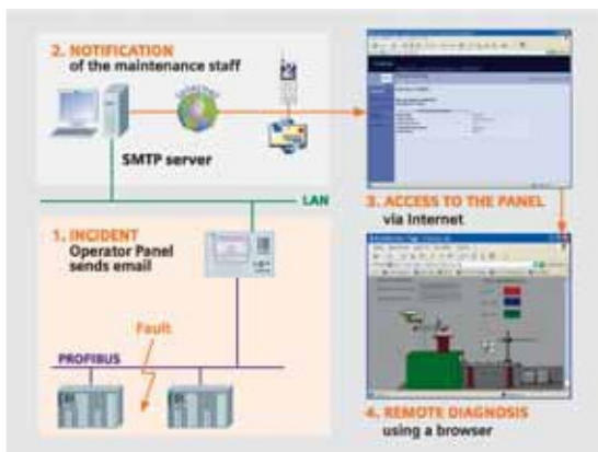
Uzaktan servis senaryosu
